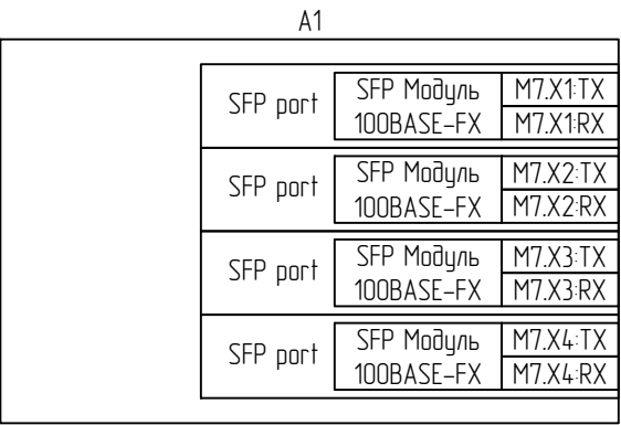
Цепи портов связи терминала
