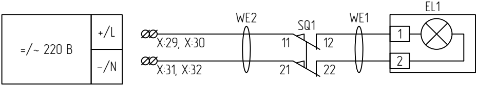
Цепи освещения шкафа
