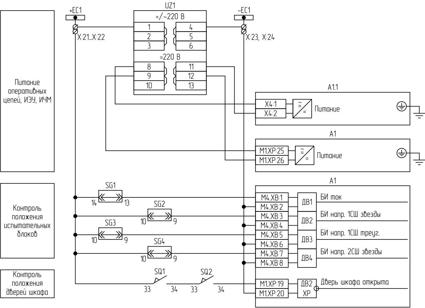
Цепи оперативного тока
