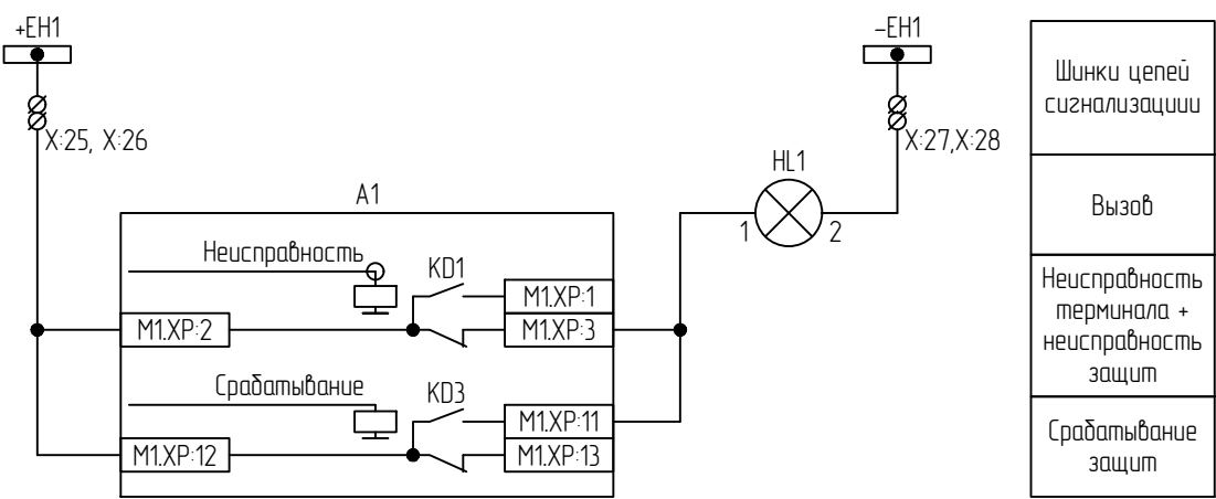
Цепи сигнализации
